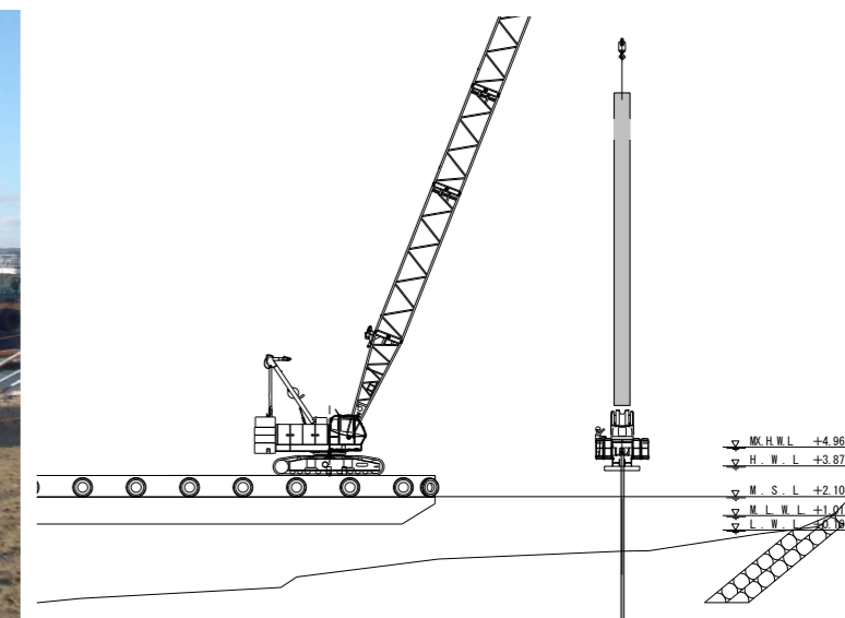
作業状況図 (鋼矢板作業イメージ)
