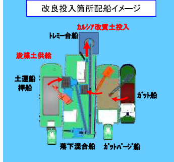
土砂改良投入作業状況図
